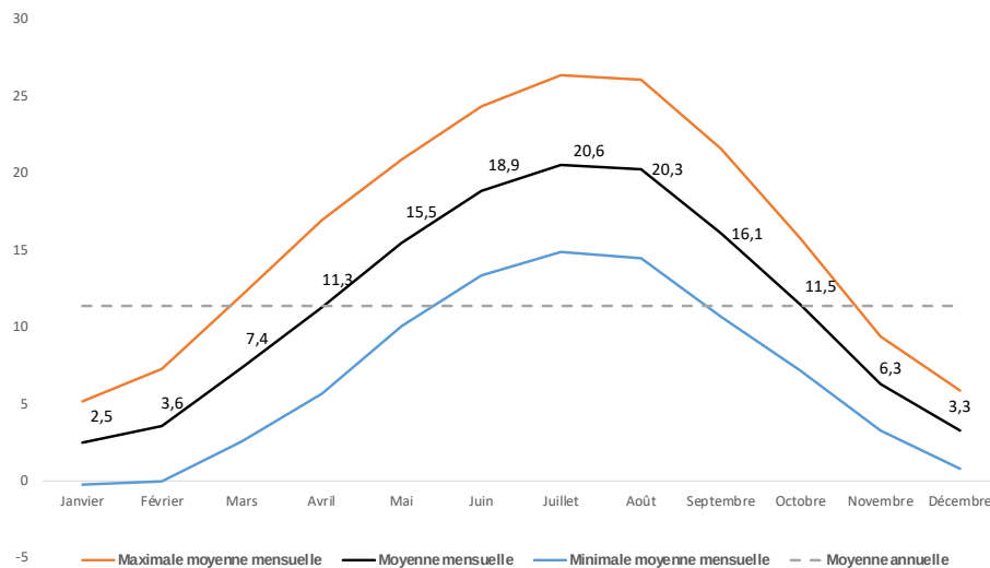
Figure 3 - Diagramme des normales de température de la station de Strasbourg-Entzheim de 1999 à 2001 (Météo France).
