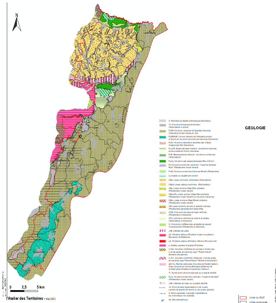
Figure 6 - Carte géologique de la bande rhénane nord (BRGM),
